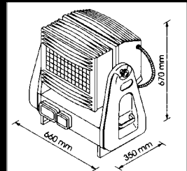
CITY COLOR 寸法図
